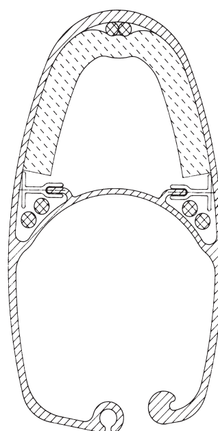
Profil: 232/126 260/136 290/150
